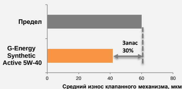
Износ деталей 1
